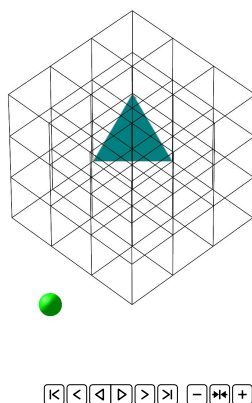
Figur 10.2: Bevægelsen af punktet w(t) i tetraederrummet. Den resulterende kurve (her en cirkel) kan betragtes som resultatet af en Cosserat-sweeping med det bevægede punkt men uden rotation og translation af tetraederrummet. Se eksempel 10.7. Hvis vi tilføjer rotation og translation får vi resultatet som vist i figur 10.3. Animeret.
