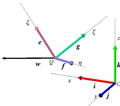
Figur 9.1: Koordinatsystemerne \{Q, \xi, \eta, \zeta\} og \{O, x, y, z\} med tilhørende basisvektorer \{e, f, g\} og \{i, j, k\} samt en vektor w med fodpunkt i Q .
