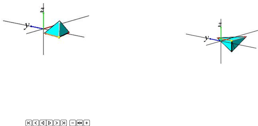
Figur 7.1: Deformation af tetraeder med \mathbf{K}(t) som specificeret i eksempel 7.4, se de definerende ligninger (7.9). Animeret.
