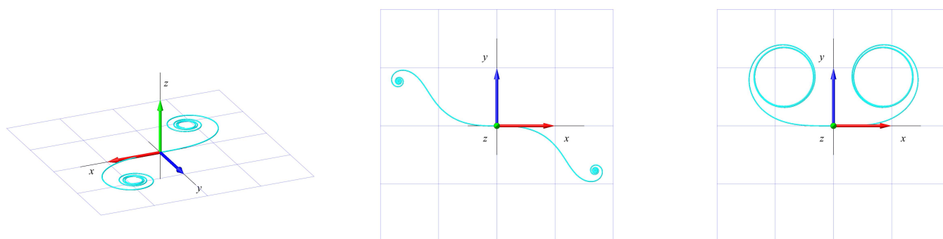
Figur 8.18: Plane kurver med givne krumningsfunktioner. Men hvilke? Se opgave 8.44.
