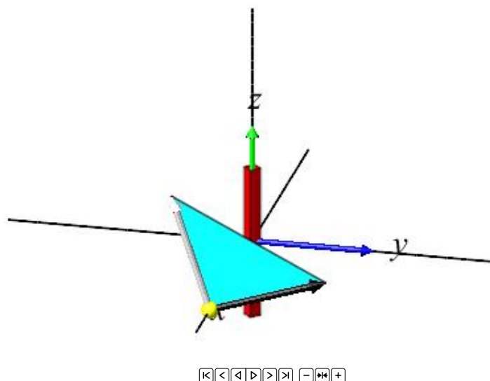
Figur 9.5: Frenet–Serret styring langs en vindellinje og den tilhørende øjeblikkelige skrue-akse. Bemærk, at \omega(t) er proportional med (0,0,1) for alle t selv om e(t) og g(t) varierer i ligning (9.55). Animeret.
